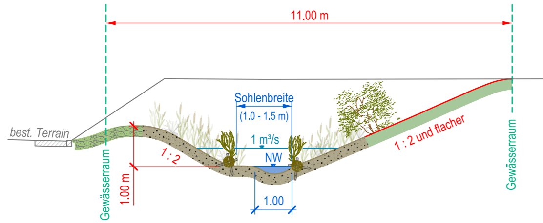
Querprofil 1
