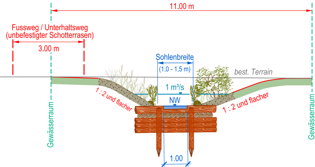
Querprofil 2
