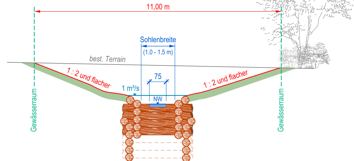
Querprofil 3
