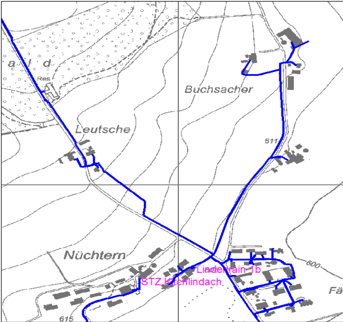
Versorgungsgebiet Transformatorstation Lindenrain 1b
